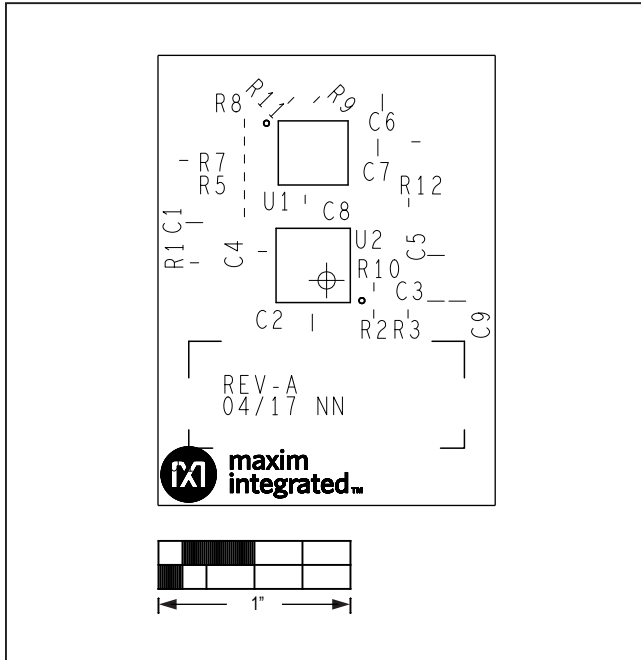
MAX86140OSBEK#—Top Silkscreen
