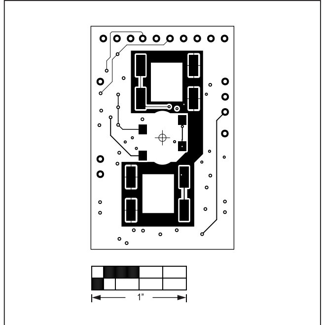
MAX86141OSBEK#—L05 SIG
