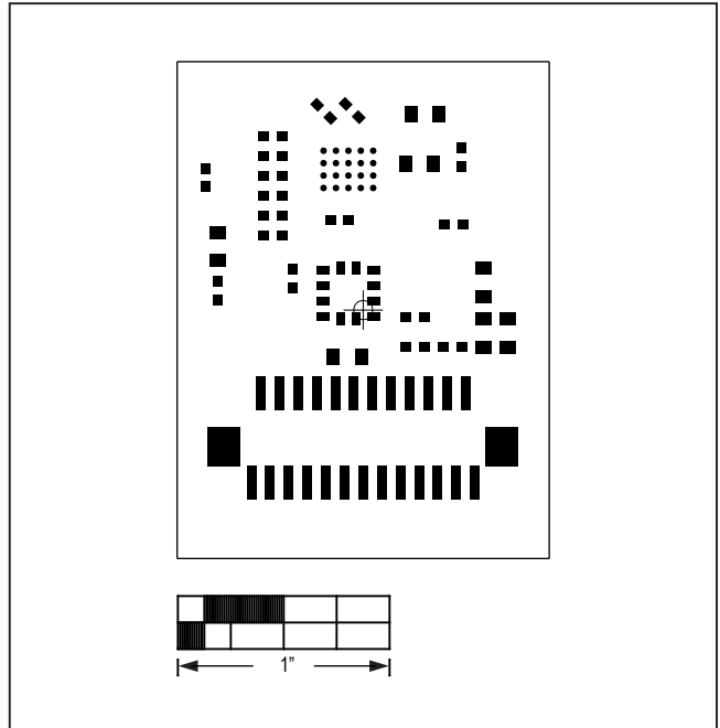
MAX86140OSBEK#—Top Paste
