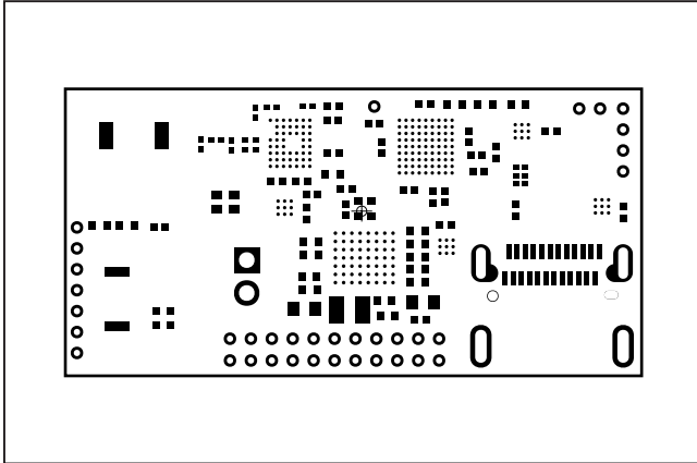
MAX32620UCBLEEK#—Top Mask
