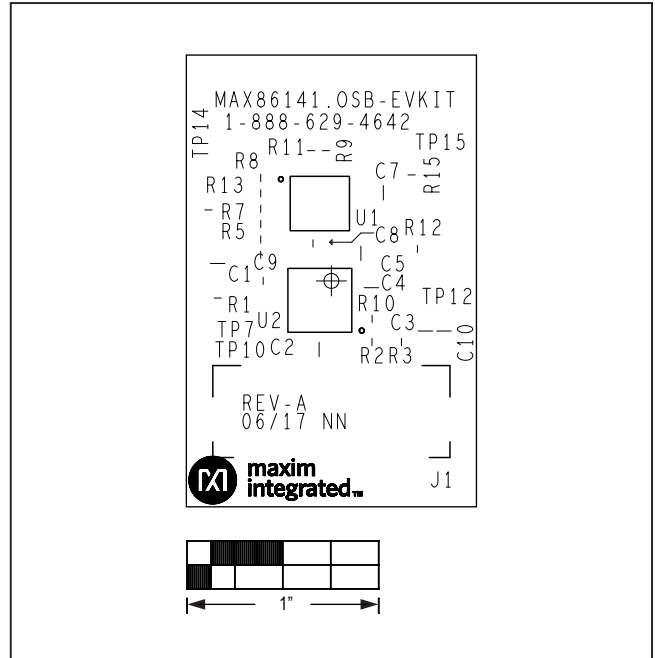
MAX86141OSBEK#—Top Silkscreen
