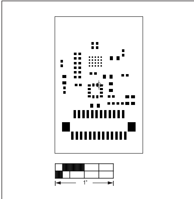
MAX86141OSBEK#—Top Paste
