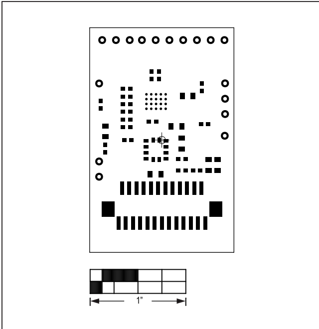
MAX86141OSBEK#—Top Mask
