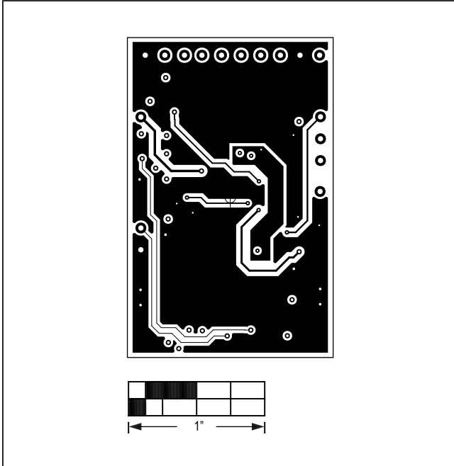
MAX86141OSBEK#—L04 SIG
