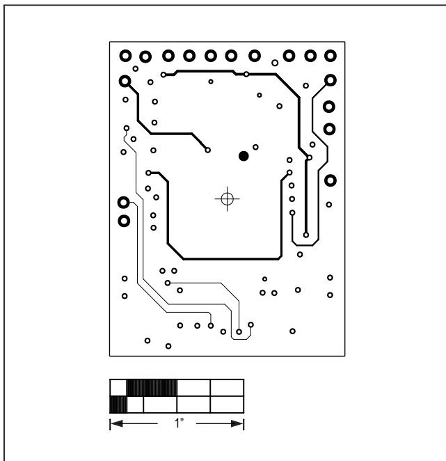
MAX86140SBEK#—L04 SIG
