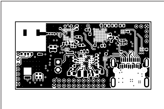
MAX32620UCBLEEK#—Top
