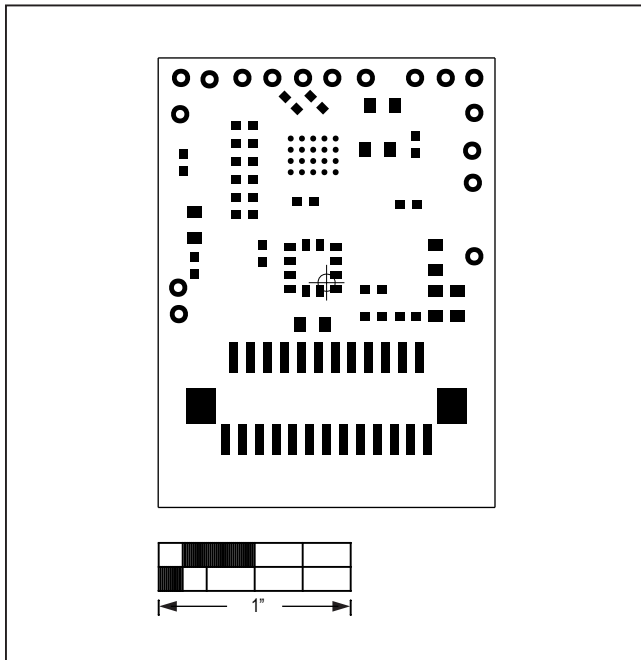
MAX86140OSBEK#—Top Mask
