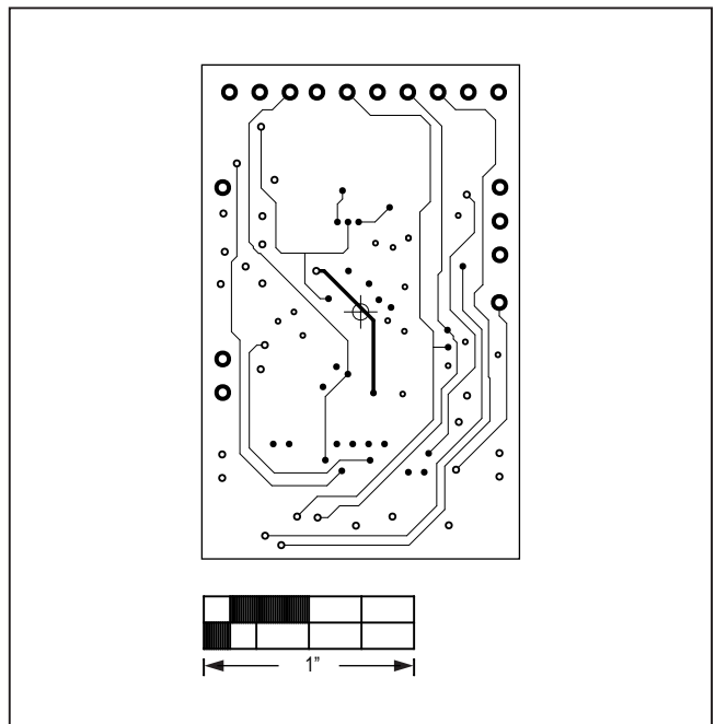
MAX86141OSBEK#—L03 SIG
