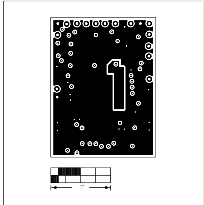
MAX86140SBEK#—L05 SIG
